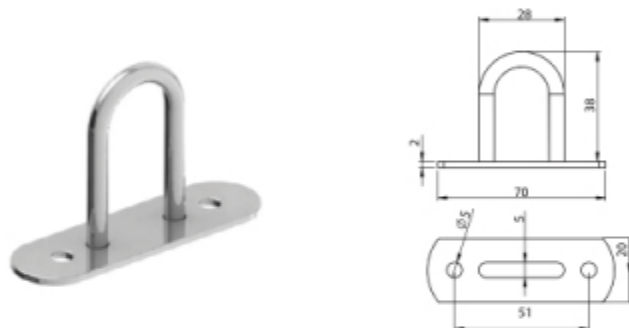
BRANDA KANCASI GALVANİZ / TARPAULIN HOOK
