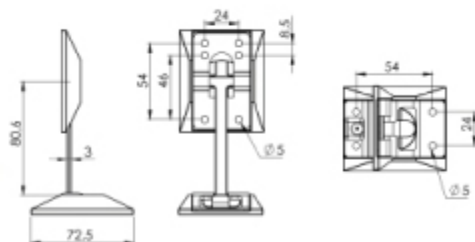
KAPI STOPU GALVANİZ - KROM / DOOR HOLDER (ZP) - (SS)
