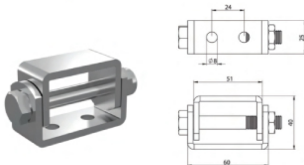
MENTEŞE GALVANİZ / HINGE
