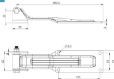
DAR MENTEŞE U AYAK KROM - DAR MENTEŞE U AYAK GALVANİZ HINGE (SS) - HINGE (ZP)
