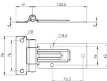
KÜÇÜK YAN KAPI MENTEŞESİ KROM - GALVANİZ SIDE DOOR HINGE (SS) - SIDE DOOR HINGE (ZP)
