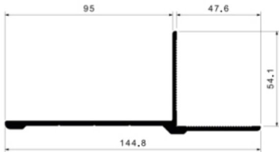
ALÜMİNYUM PROFİL / ALUMINIUM PROFILE
